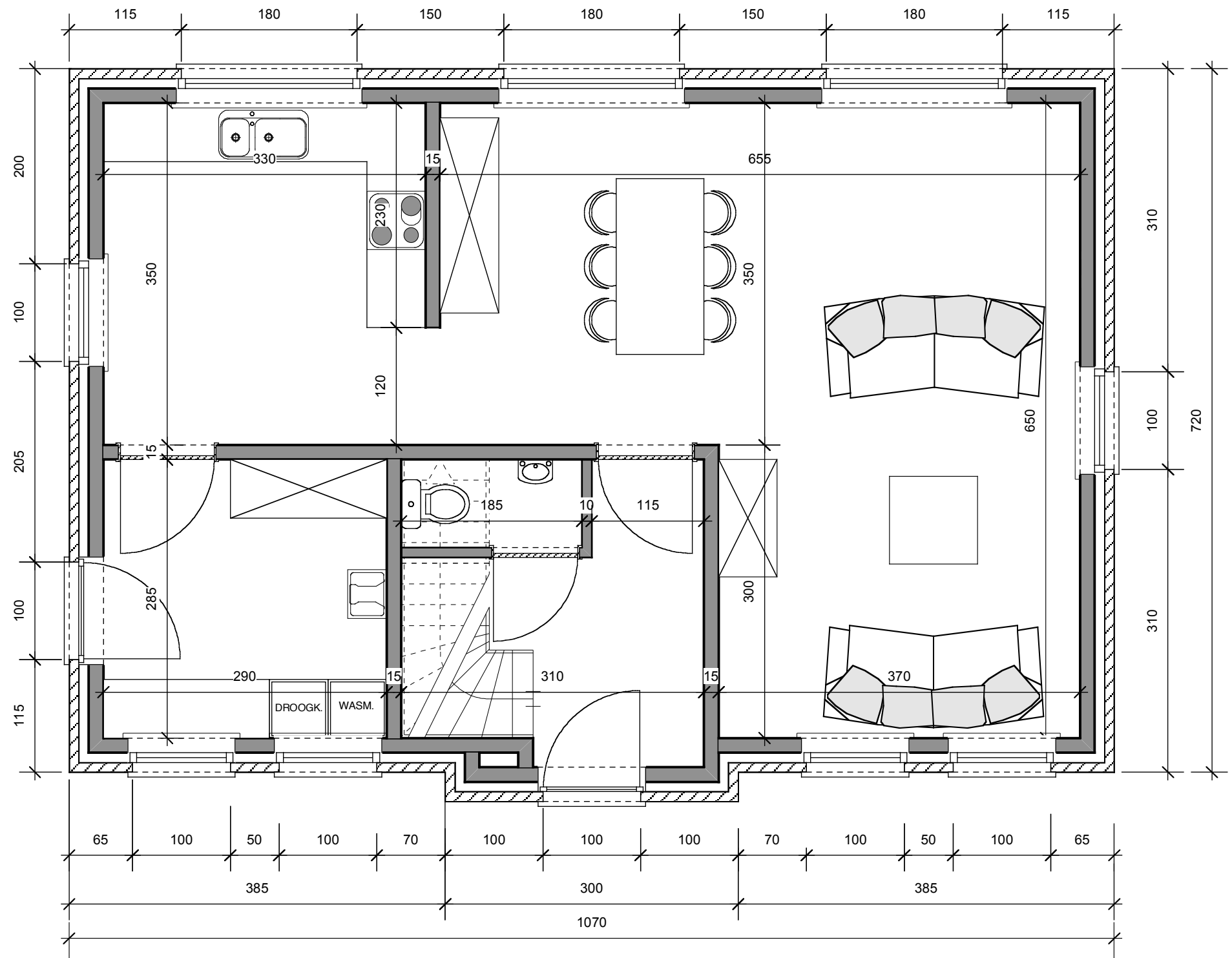
GELIJKVLOERS
