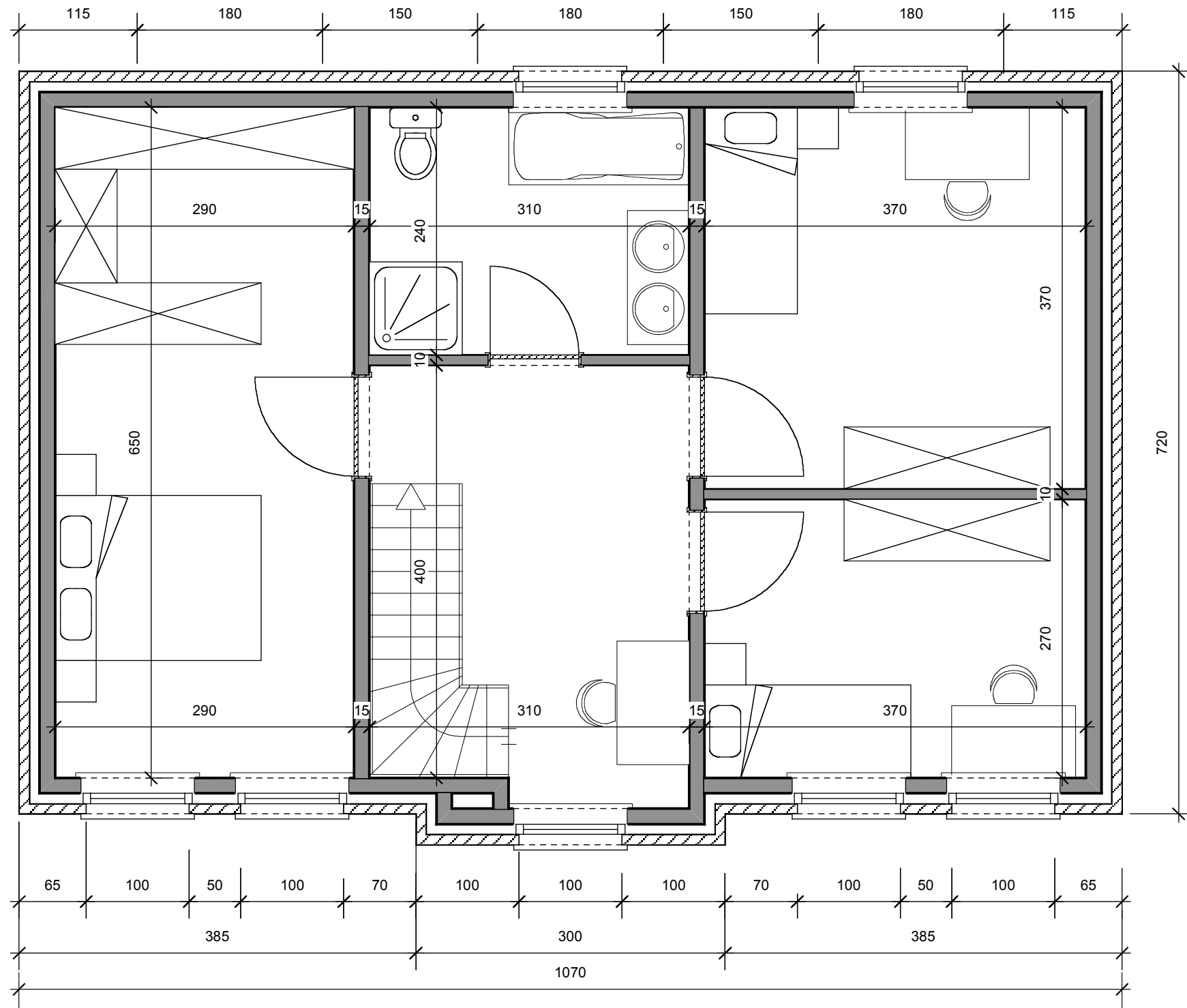
VERDIEPING
