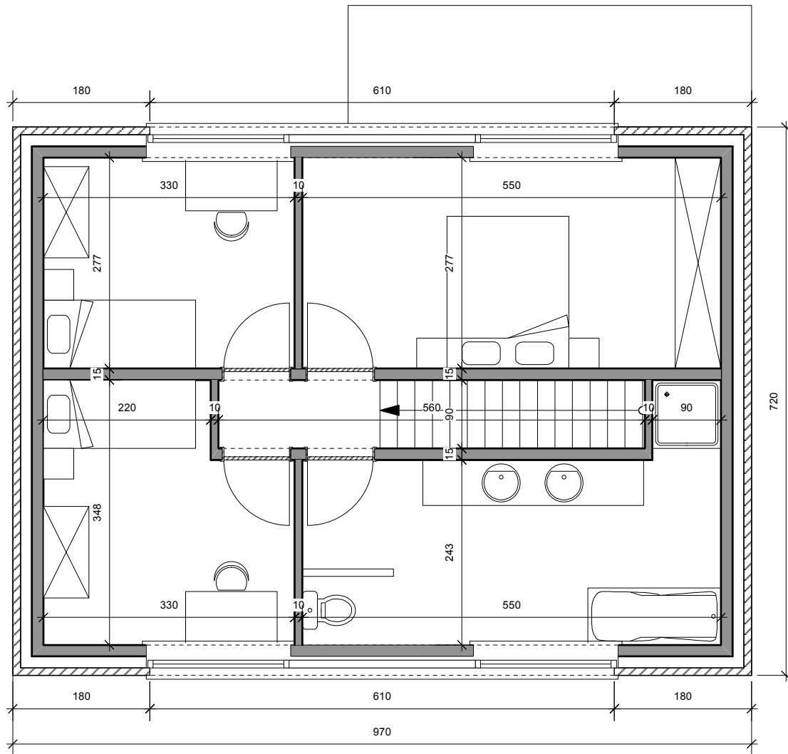
VERDIEPING
