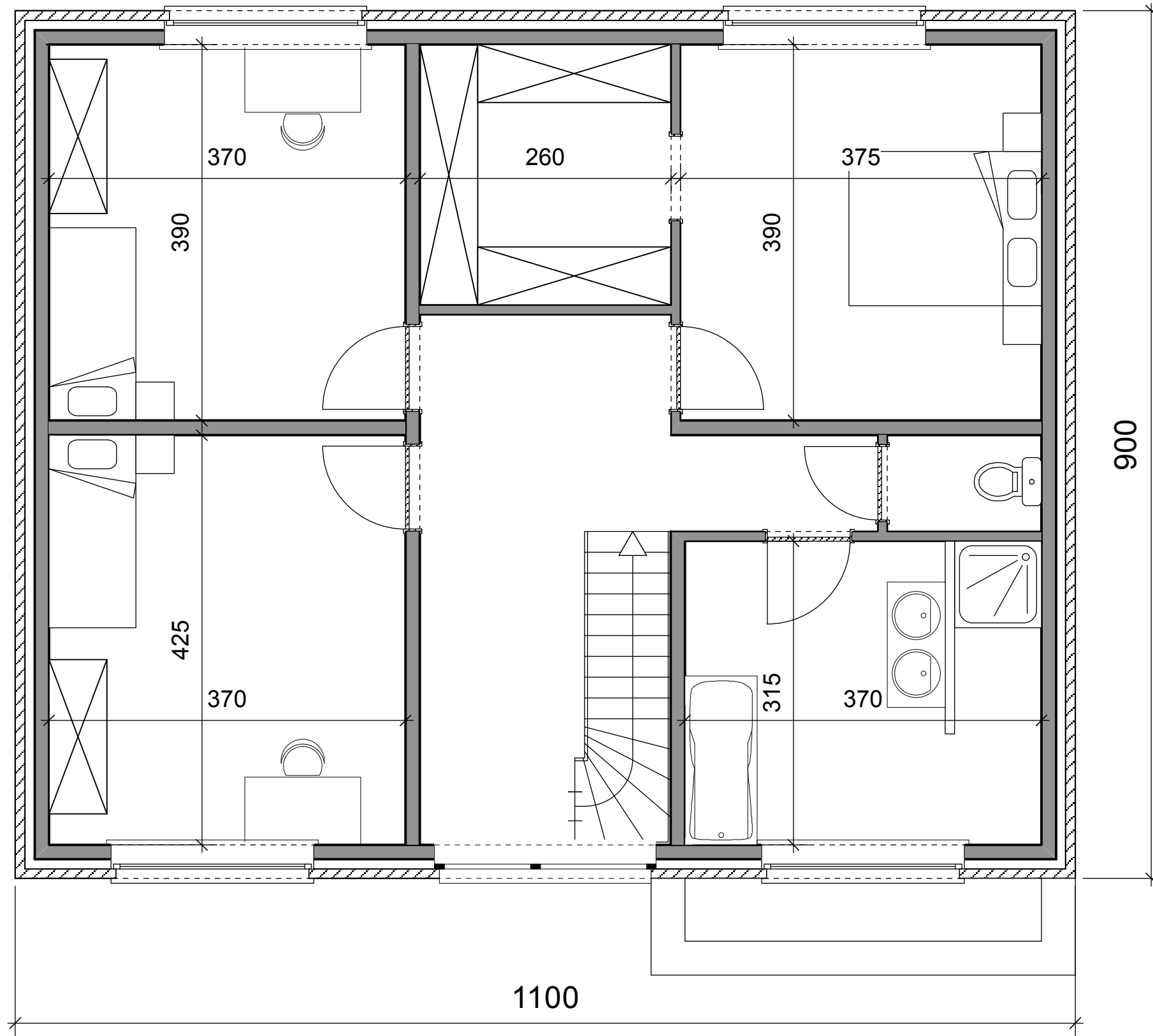
VERDIEPING
